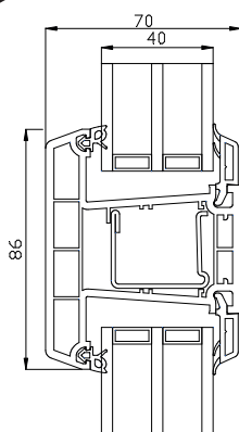
Querprofil
