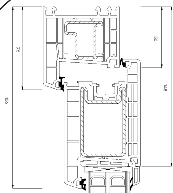
Oberer Türrahmen
