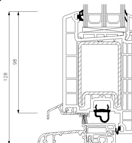
Türschwelle
