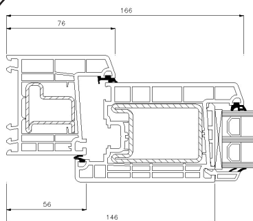
Seitenrahmen
