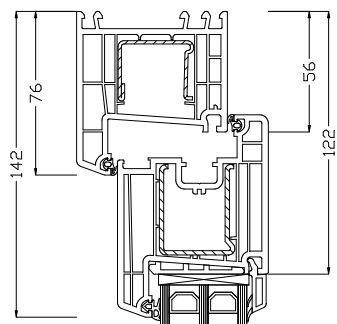
Oberer Türrahmen
