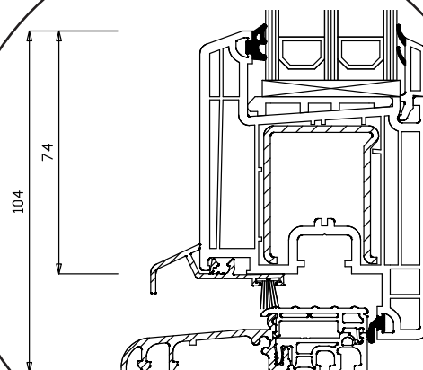
Türschwelle
