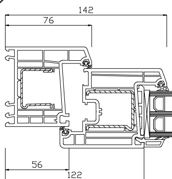
Seitenrahmen
