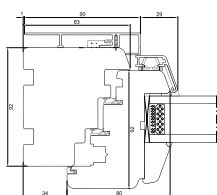
Seitenrahmen
